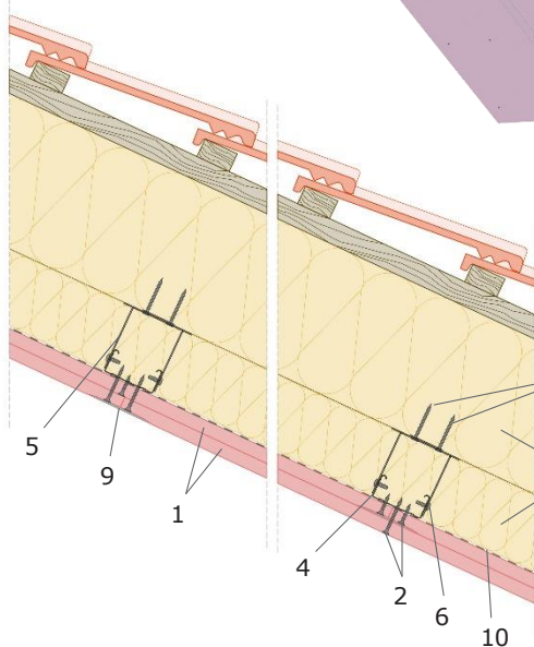
Secțiune transversală:
