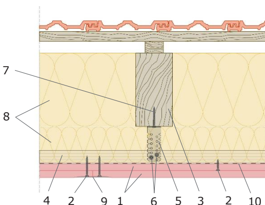
Secțiune longitudinală:
