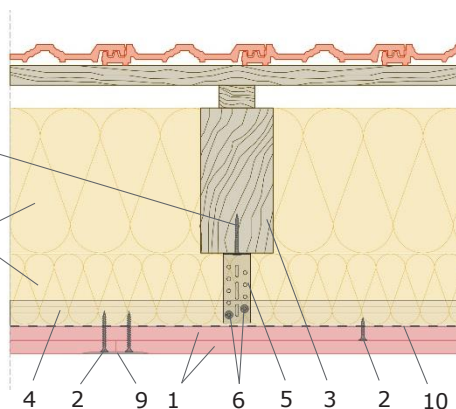
Secțiune longitudinală:
