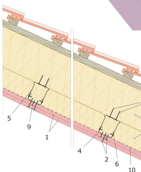
Secțiune transversală:
