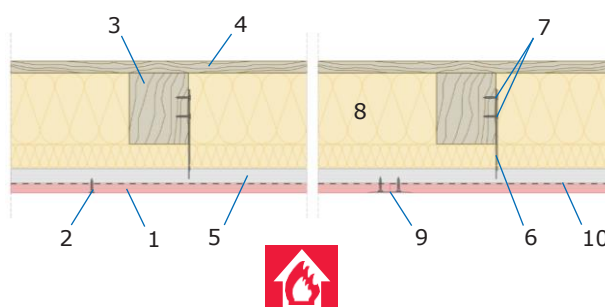
Secțiune B-B:
