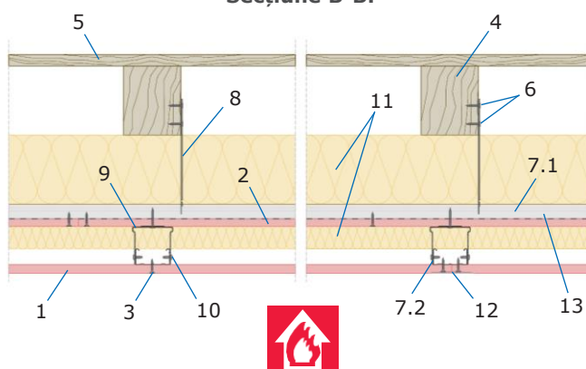
Secțiune B-B:
