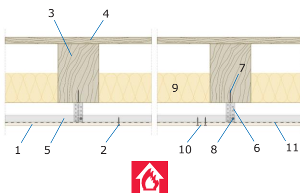
Secțiune B-B:
