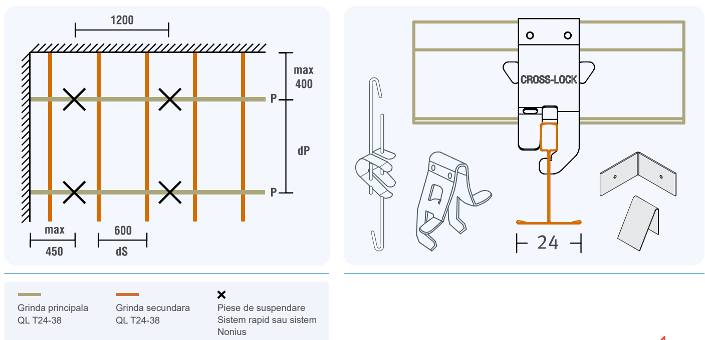
sistem D2 - structura ascunsă, plăci 600 x 600 mm muchie D2, montaj pe structură Quick-Lock® Cross-Lock T24-38
