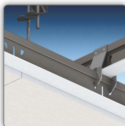
sistem D2 plăci Gyptone® muchie D2 montate pe structură Quick-Lock® Cross-Lock T24-38 sistem cu structură ascunsă
