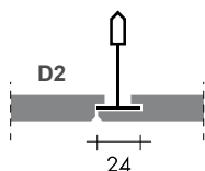
muchie D2 - structură ascunsă
