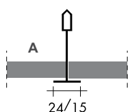
muchie A - structură vizibilă
