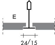
muchie E - structură retrasă
