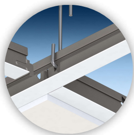
sistem Quick-Lock® structură retrasă
