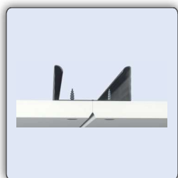
sistem B - CD plăci cu muchie B montate pe structură CD 60, sistem nedemontabil, structură ascunsă, fixare cu șuruburi
