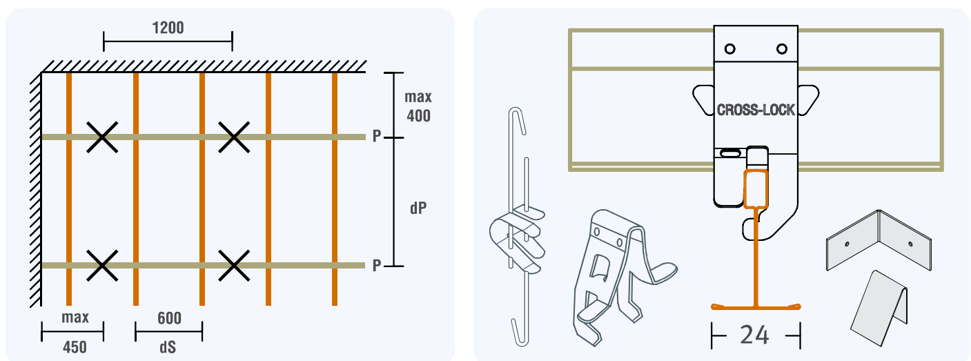
sistem D2 - structura ascunsă, plăci 600 x 600 mm muchie D2, montaj pe structură Quick-Lock® Cross-Lock T24-38
