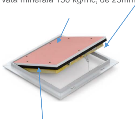
garnitură termosupantă pe conturul foii mobile (neagră)
