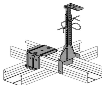
DETALIU sistem Nonius & piesă de încrucișare CD 60
