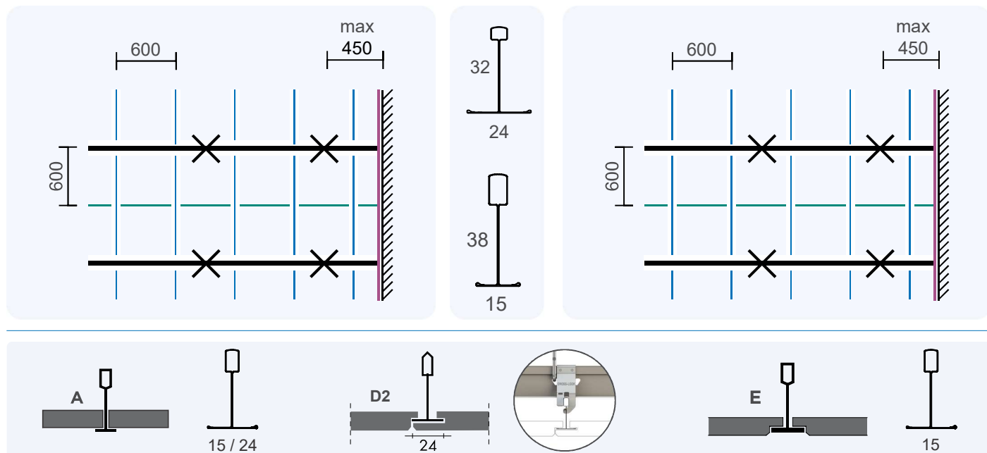
sistem A - plăci muchie A modul standard 600 x 600 mm
