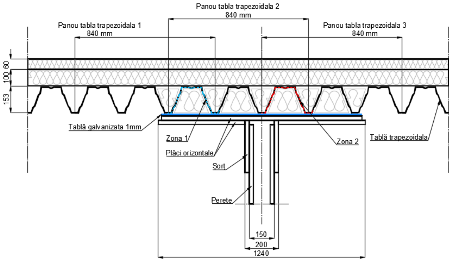
LJ2. RF HL M2 b. Ax perete centrat pe mijlocul vutei inferioare cu 2 zone de suprapunere ale vutelor
