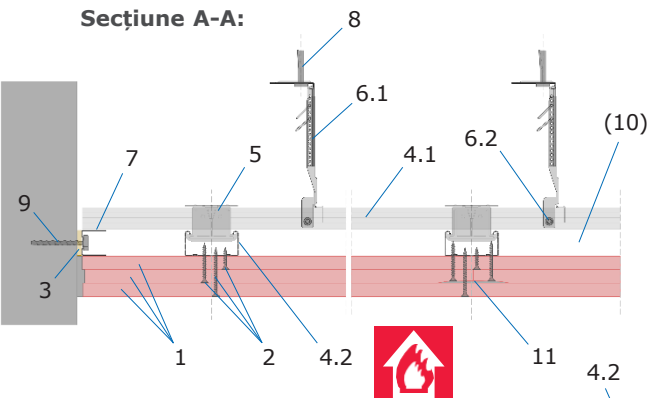
Secțiune A-A:
