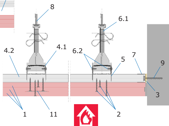
Secțiune B-B:
