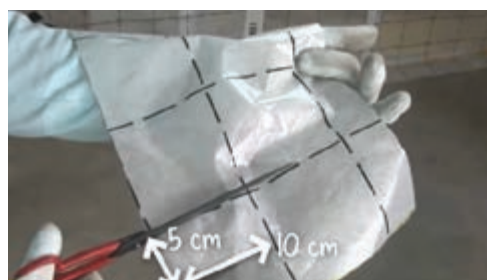
Figura 48. Decuparea bucății de membrană pentru etanșarea străpungerii cu o tubulatură
