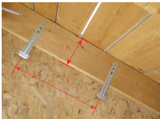
Figura 7. Distanța între ancore pe un căprior și înălțimea căpriorului
