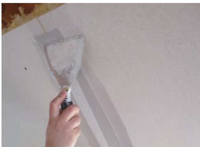
Figura 68. Aplicarea benzii de armare la îmbinarea dintre plăcile din gips-carton
