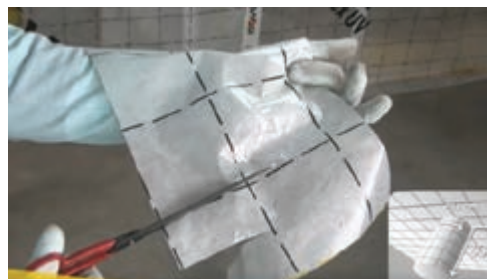
Figura 47. Decuparea bucății de membrană pentru etanșarea străpungerii cu o tubulatură
