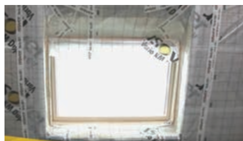
Figura 45. Golul ferestrei de mansardă după aplicarea membranei ISOVER Vario® KM Duplex UV
