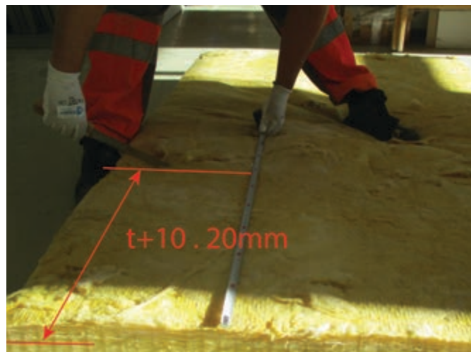
Figura 15. Tăierea unei bucăți de vată minerală pentru stratul dintre căpriorii unei zone de acoperiș
