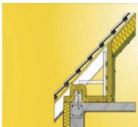
Figura 25. Stratul de vată minerală în spatele zonei de placare verticală
